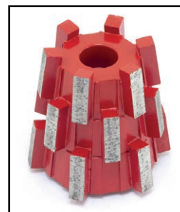
Fraise tronconique avec segments H1
